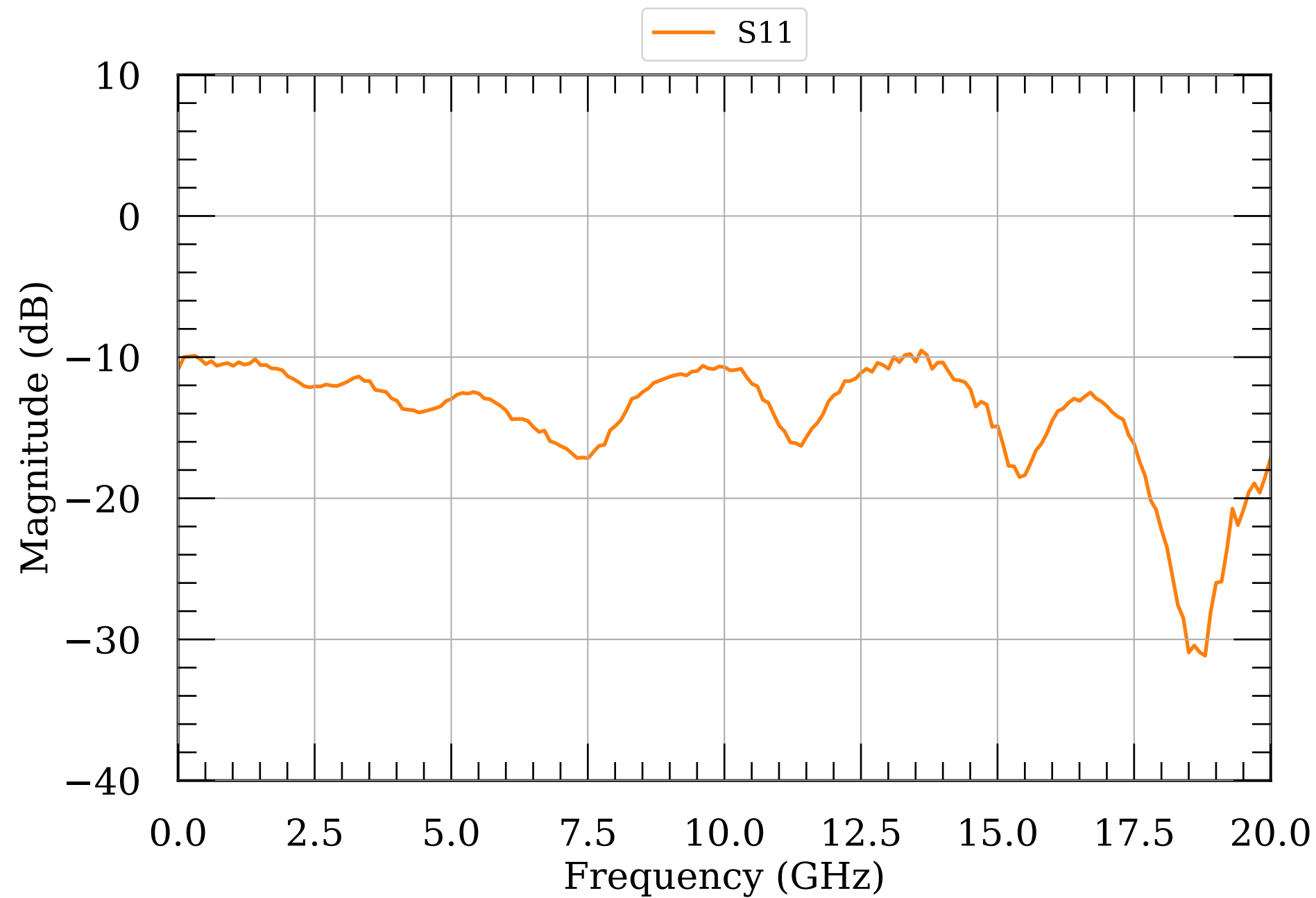
LNA S-params module049
